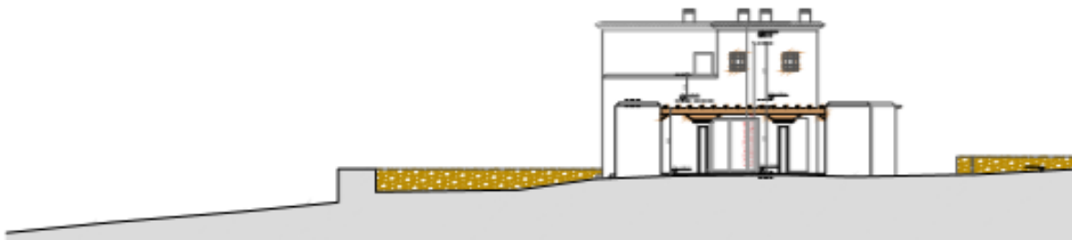
ALZADO NOR-ESTE escala 1/100
