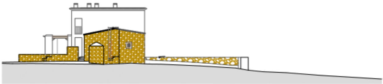
ALZADO NOR-ESTE escala 1/100
